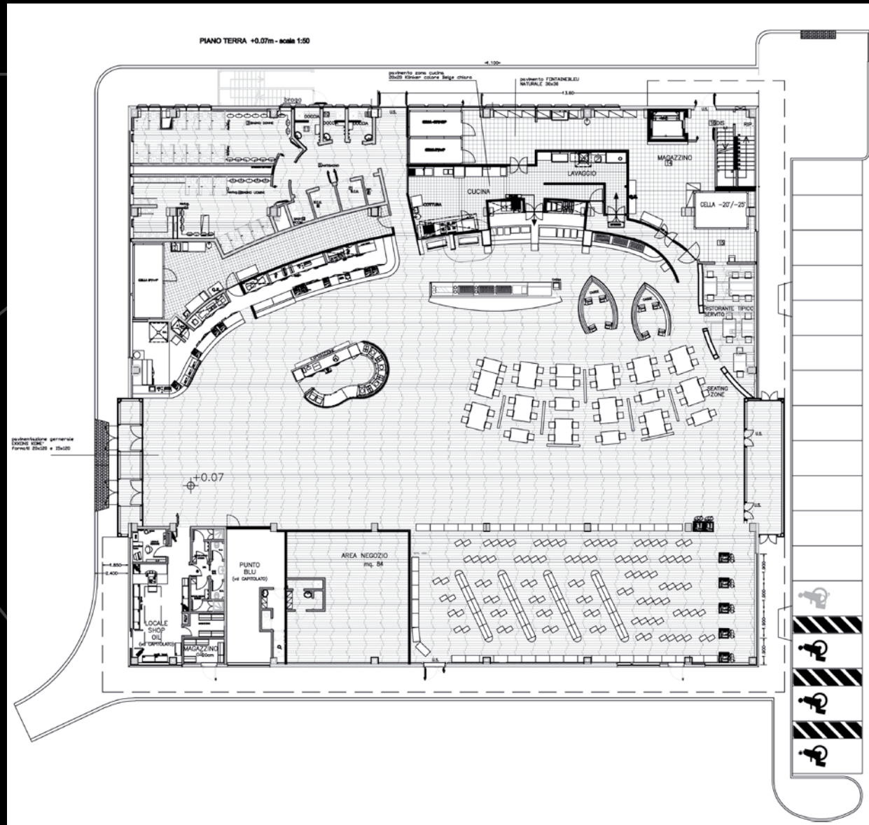
STUDIO DI PROGETTO CON APPREDI: pianta
