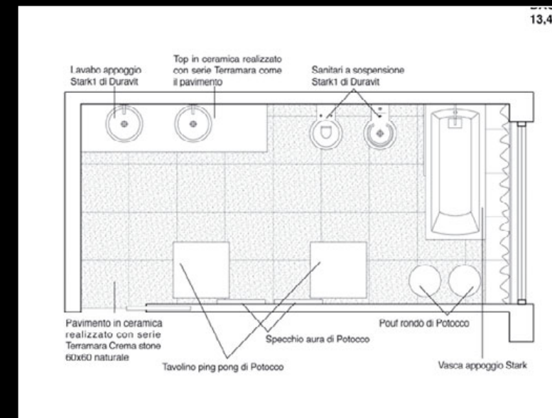
STUDIO DI PROGETTO CON ARREDI: pianta
